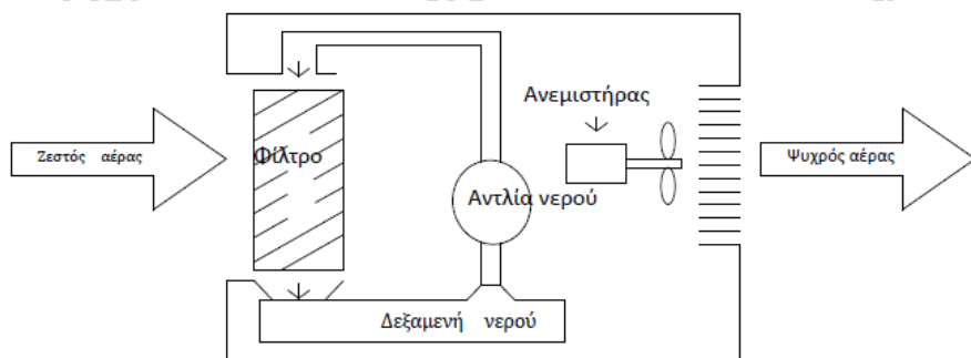
Βασικό διάγραμμα
