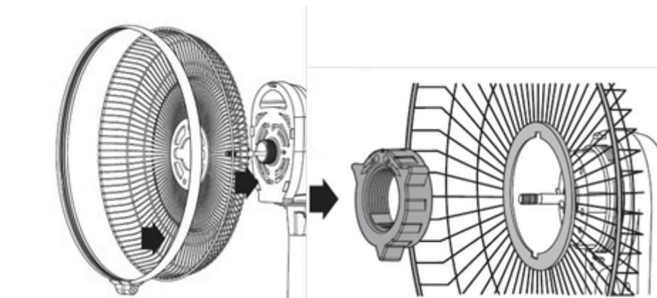
Εικ. 1 – Τοποθέτηση ωτίδων και παξιμαδιών ασφάλισης
